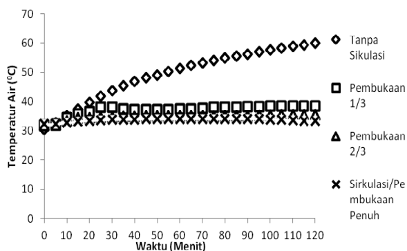
Gambar 11. Temperatur air ditangki kondensator dummy pada pembukaan katup
