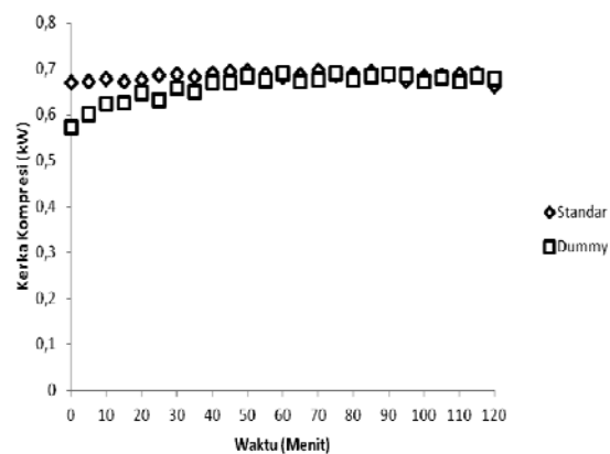
Gambar 8. Perbandingan kerja kompresi standar dan penambahan dummy
