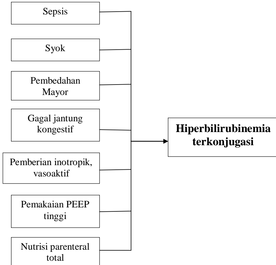
Gambar 2. Kerangka Konsep
