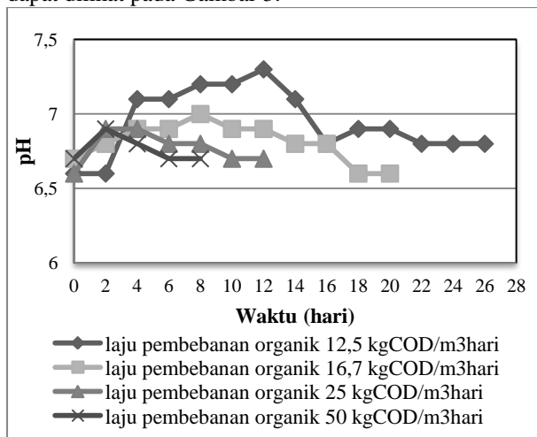
Gambar 3. Perubahan pH Selama Transien
