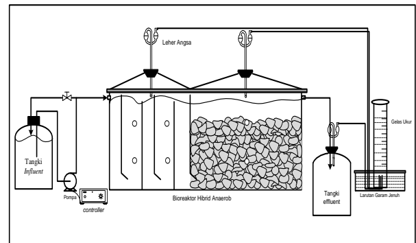
Gambar 2. Rangkaian Peralatan Pengolahan dengan Menggunakan Bioreaktor Hibrid Anaerob Bermedia Batu
