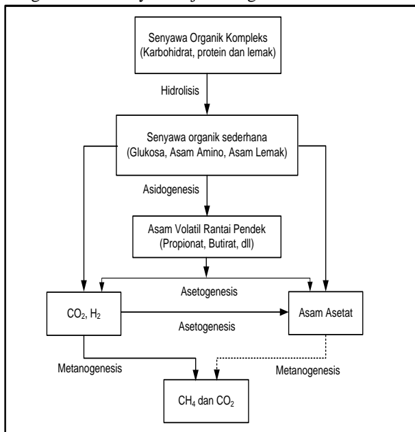
Gambar 1. Lintasan Biodegradasi Zat Organik Kompleks dalam Proses Anaerob [Pavlostathis dan Giraldo-Gomez, 1991]
