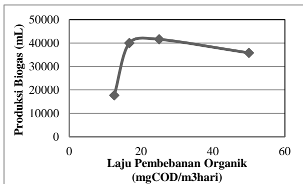
Gambar 5. Pengaruh Laju Pembebanan Organik terhadap Produksi Biogas
