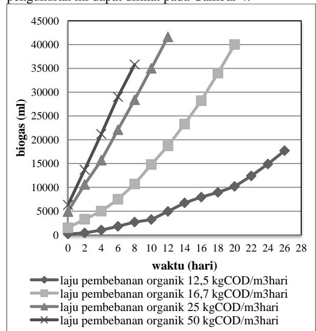
Gambar 4. Produksi Biogas Selama Transien
