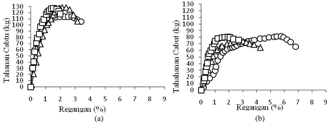
Gambar 3 Tahanan cabut perkuatan bentuk (a) persegi tunggal, (b) segi tiga
