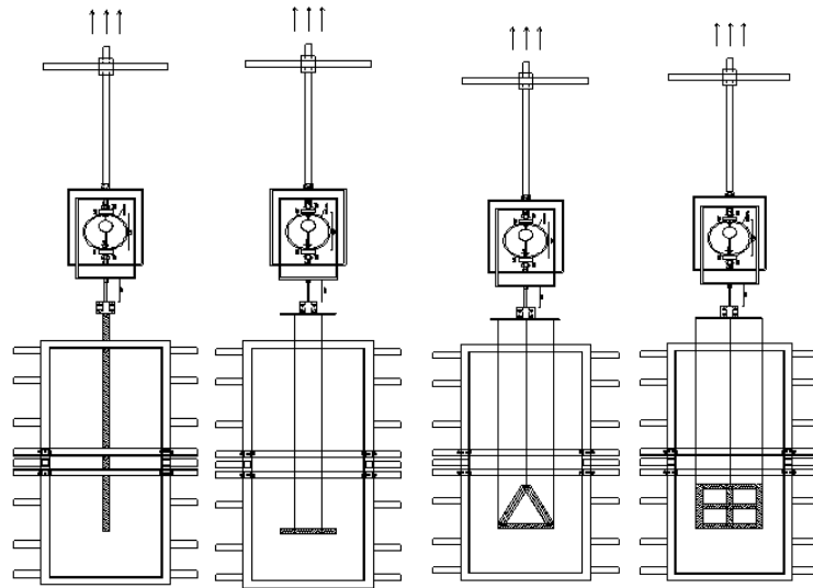
Gambar 1. Kotak uji perkuatan cabut dan bentuk perkuatan
