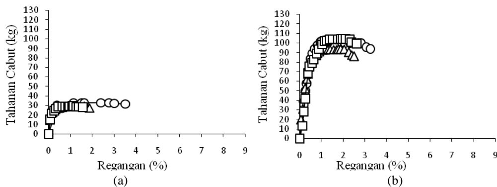
Gambar 2 Hubungan waktu terhadap tahanan cabut (a) arah longitudinal (b) transversal
