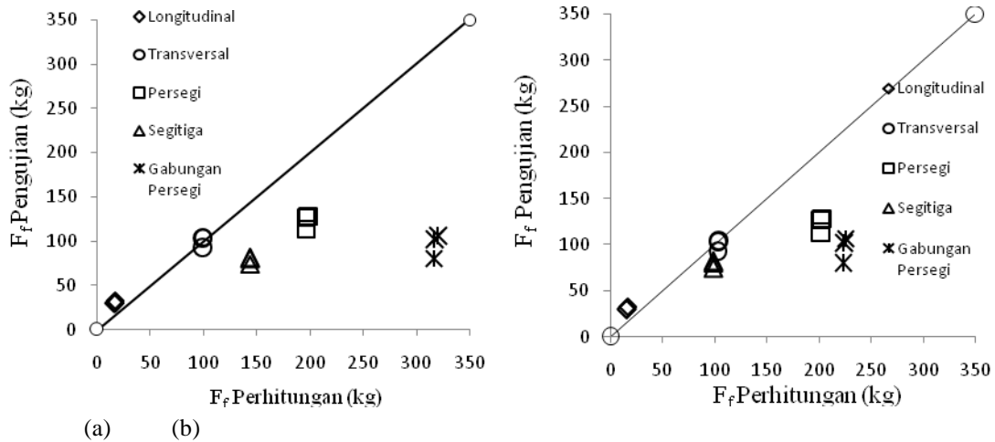
Gambar 5. Perbandingan tahanan cabut secara pengujian dengan pengukuran (a) menurut Kwon, 2010 (b) Braja M. Das, 1993.
