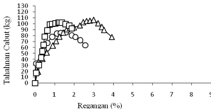
Gambar 4. Tahanan cabut perkuatan berbentuk gabungan persegi
