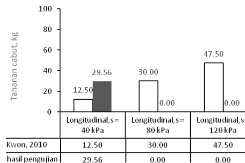
Gambar 7 Perbandingan tahanan cabut hasil studi dengan hasil pengujian Kwon (2010)
