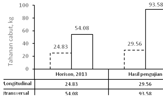
Gambar 6 Perbandingan tahanan cabut hasil studi dengan hasil pengujian Harison (2013)
