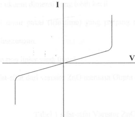
Gambar 1. Pola Hubungan Arus I dan Tegangan V pada Varistor (Moulson A.J. and Herbert J.M. 1990).
