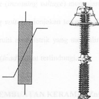
Gambar 4. Varistor ZnO yang digunakan di jaringan listrik tegangan tinggi sebagai Switchgear (Mattias E, 2002).
