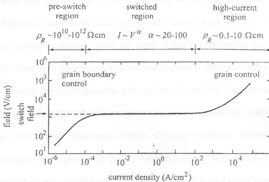
Gambar 2. Kurva hubungan arus I dengan tegangan V dari Varistor ZnO (Gupta 1991, Mattias E, 2002)
