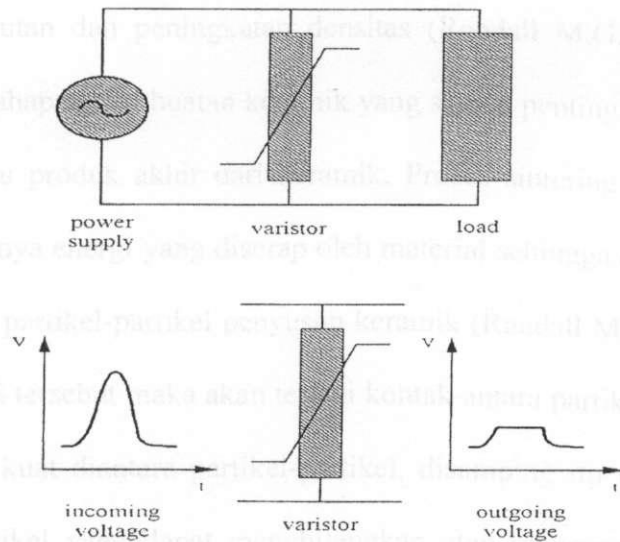
Gambar 5. Skema rangkaian aplikasi varistor (Mattias E, 2002).
