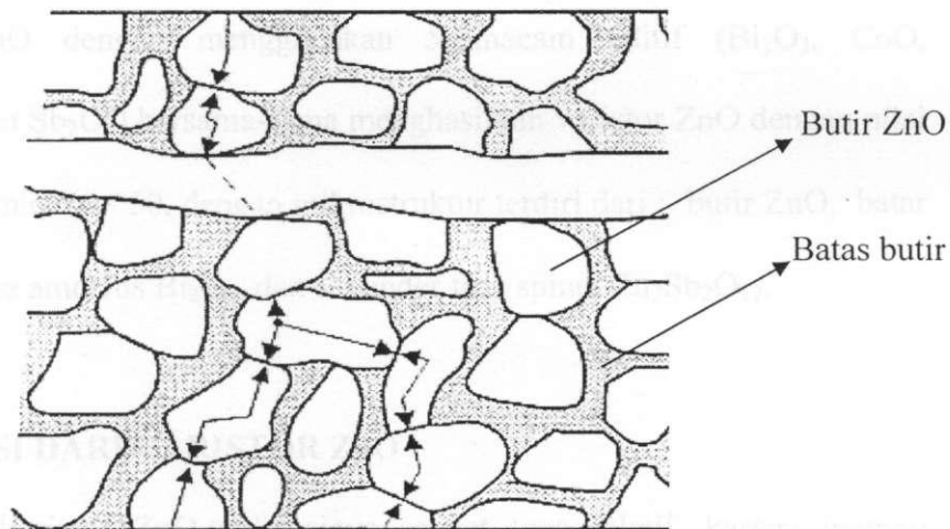
Gambar 3. Mikrostruktur dari ZnO.
