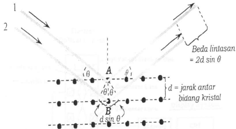
Gambar 9. Difraksi Dari Bidang Kristal
