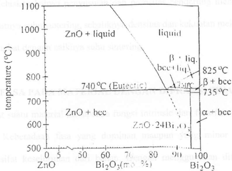
Gambar 7. Diagram fasa sistem biner dari ZnO - Bi 2 O 3 (Mattias E, 2002).
