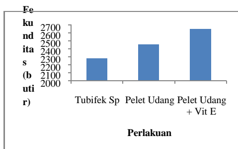
Gambar 5. Histogram nilai fekunditas
