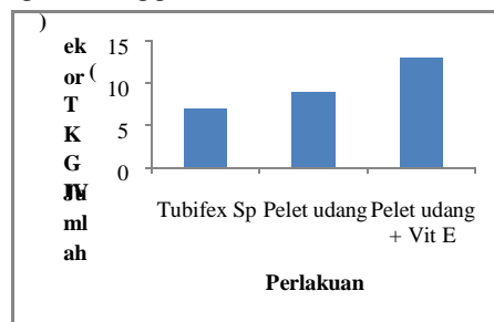
Gambar 2. Histogram jumlah ikan
