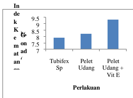
Gambar 4. Histogram nilai rata-rata indeks kematangan gonad (%) ikan sepat mutiara pada masing-masing perlakuan.
