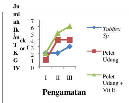
Gambar 3. Grafik ikan sepat mutiara yang mencapai TKG IV dari pengamatan sampai pengamatan ke III.
