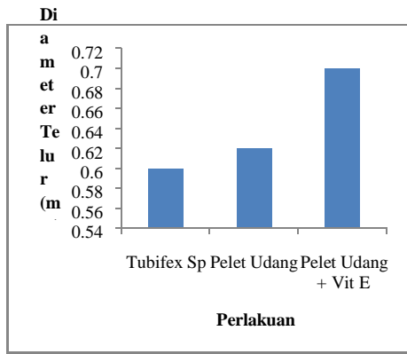
Gambar 6. Histogram rata-rata diameter telur ikan sepat mutiara pada setiap perlakuan.
