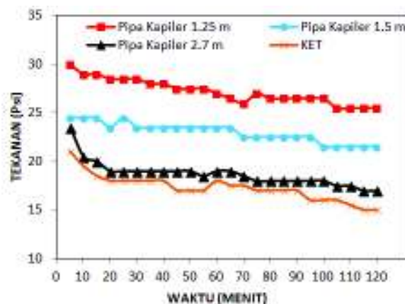
Gambar 9. Perbandingan Tekanan pada Evaporator
