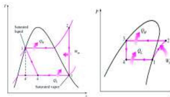
Gambar 2. Diagram 1-s dan P-h Siklus Kompresi Uap [5]
