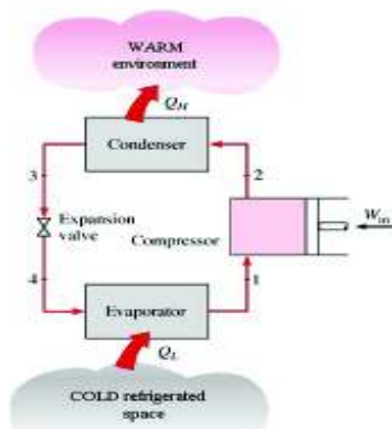
Gambar 1. Mesin Refrigerasi Siklus Kompresi Uap [5]
