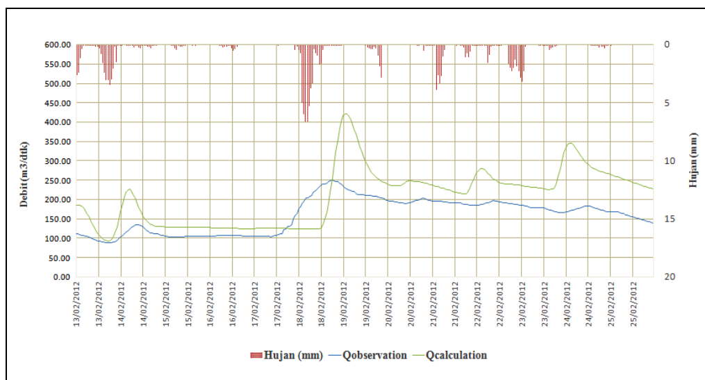
Gambar 5 Hidrograf hasil simulasi pada kondisi awal sebelum kalibrasi (13 - 25 Februari 2012) di Stasiun Lubuk Bendahara
