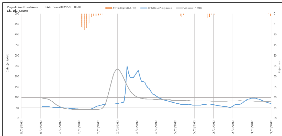
Gambar 8. Perbandingan hidrograf hasil simulasi dengan data terukur dari AWLR Stasiun Pasir Pangaraian setelah kalibrasi
