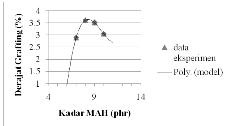
Gambar 3. Perbandingan kadar MAH dengan derajat grafting pada suhu 160°C berdasarkan persamaan polinomial
