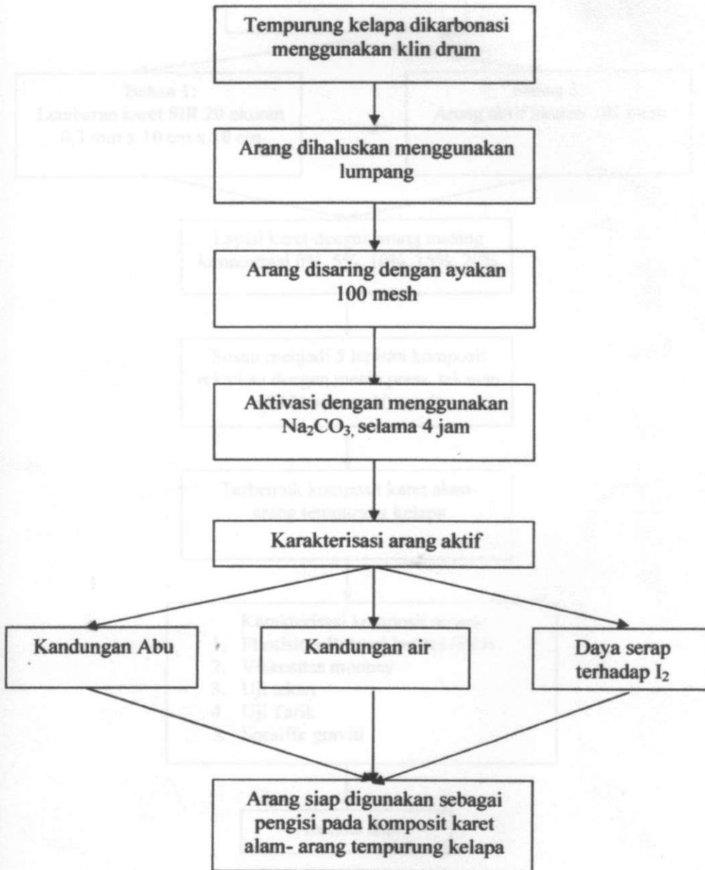
Gambar 10. Pembuatan komposit karet alam- arang aktif tempurung kelapa 100 mesh
