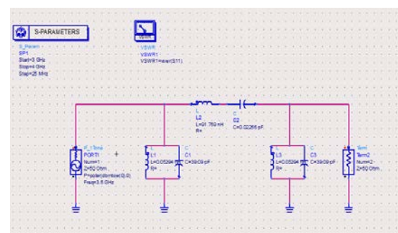
Gambar 11. Band pass Filter dalam ADS
