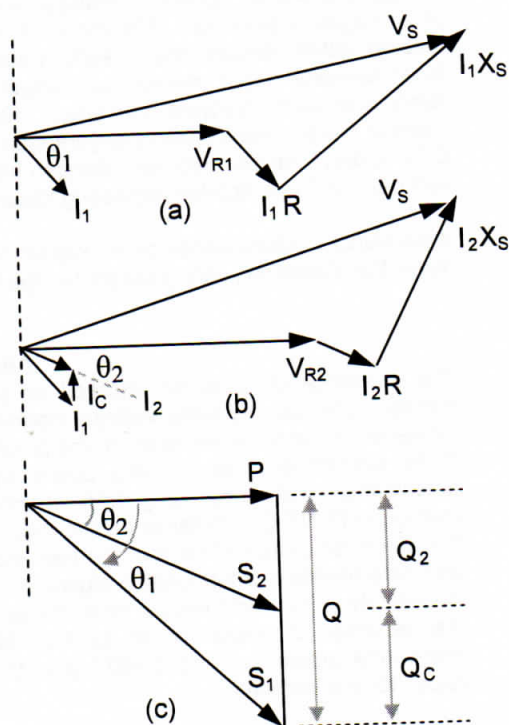
Gambar 1. Diagram fasor kondisi jaring sistem tenaga listrik sebelum dan sesudah penambahan kapasitor paralel. (a). Sebelum penambahan (b). Sesudah penambahan (c). Komposisi Segitiga Daya
