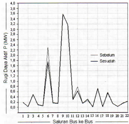
Gambar 6. Grafik kondisi daya aktif P
