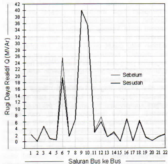
Gambar 7. Grafik kondisi daya reaktif Q
