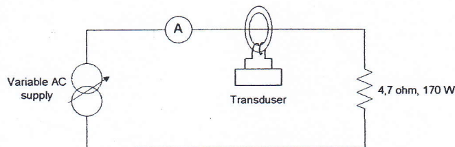
Gambar 8. Rangkaian pengujian
