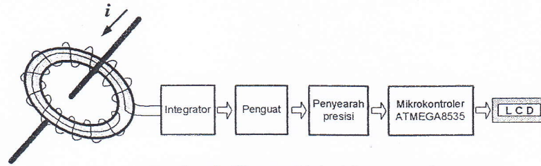
Gambar 2: Diagram blok sistem pengukuran
