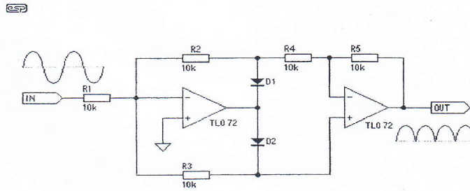
Gambar 5. Rangkaian penyearah presisi [11]
