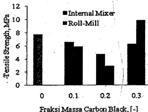
Gambar 1. Pengaruh komposisi CB terhadap sifat kuat tarik untuk teknik pencampuran berbeda
