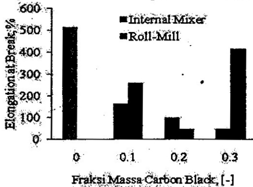
Gambar 2. Pengaruh komposisi CB terhadap sifat elongation at break untuk teknik pencampuran berbeda
