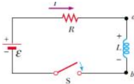
Gambar 1. Skema rangkaian RL
