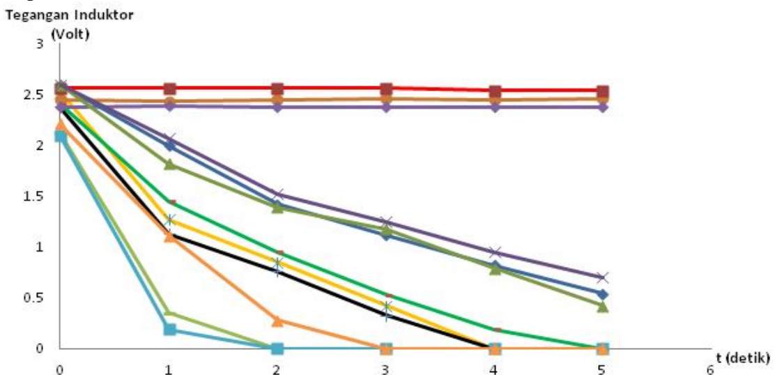
Gambar 6. Tegangan Induktor sebagai fungsi waktu (t) untuk koil tanpa inti dan koil dengan inti Fe, Al, dan Cu
