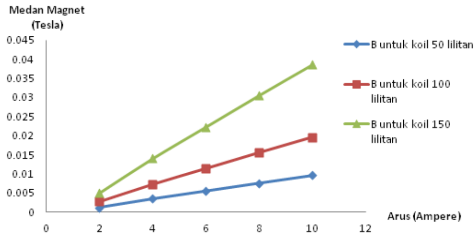
Gambar 3. Medan magnetik (T) sebagai fungsi arus
