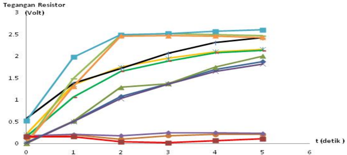
Gambar 7. Tegangan resistor sebagai fungsi waktu (t) untuk koil tanpa inti dan koil dengan inti Fe, Al, dan Cu
