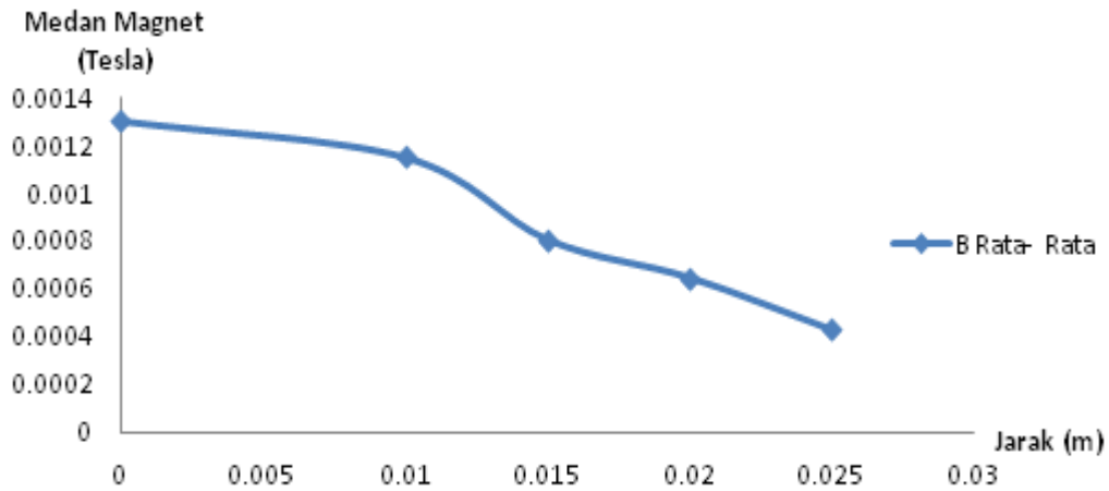
Gambar 4. Hubungan jarak terhadap besar medan magnet
