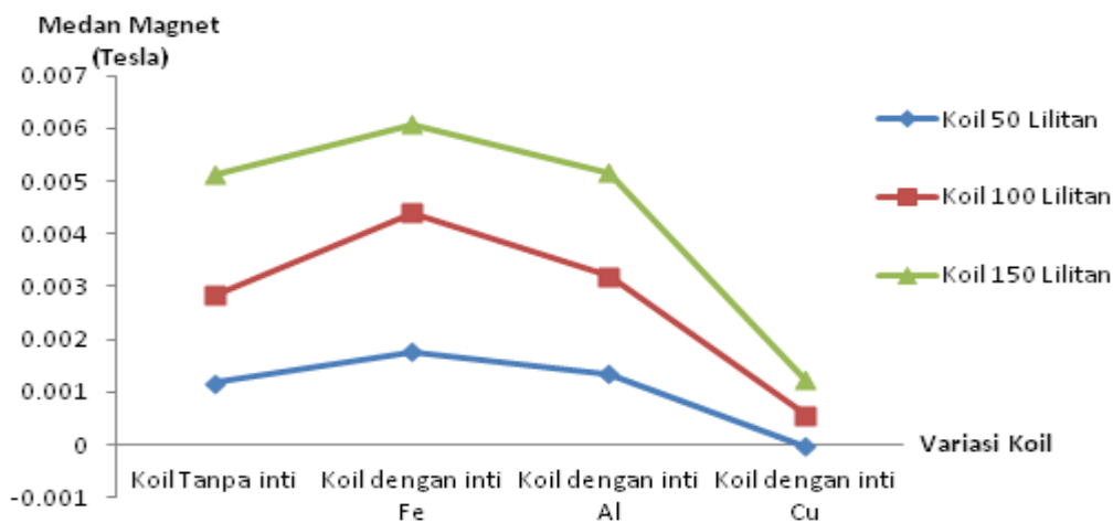
Gambar 5 Pengaruh inti terhadap medan magnet pada koil
