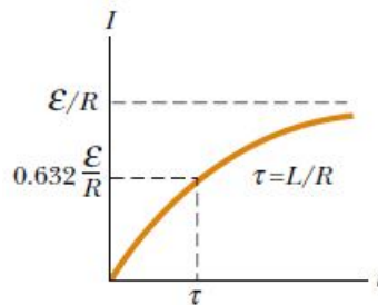
Gambar 2 Respon transien rangkaian RL
