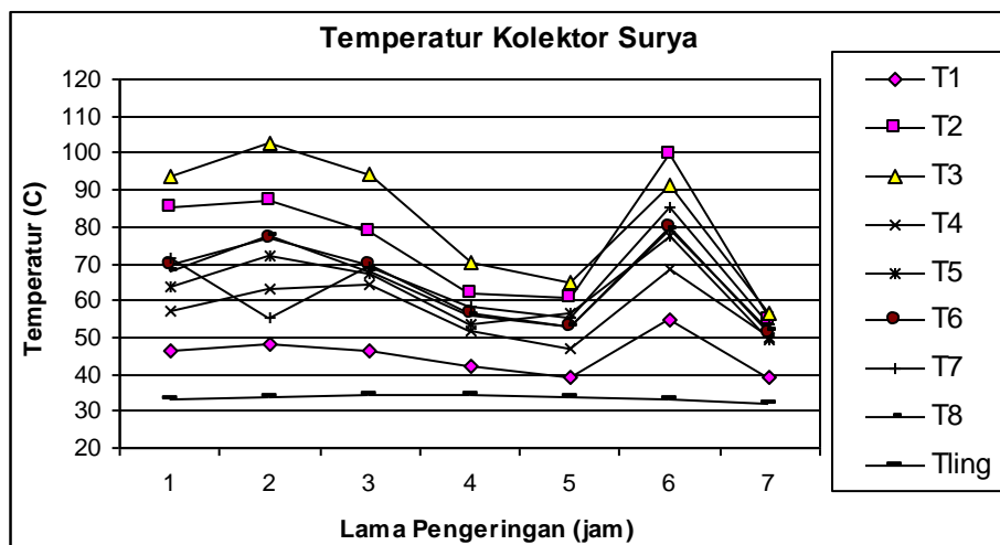
Gambar 3. Distribusi temperatur pengeringan hari 2
