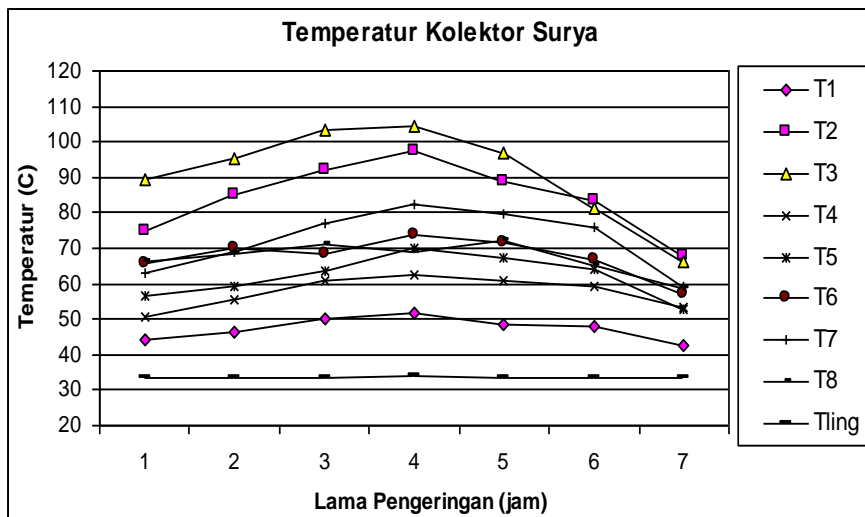
Gambar 2. Distribusi temperatur pengeringan hari 1
