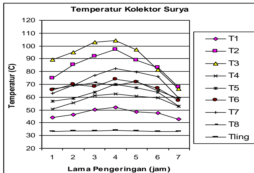
Gambar 4.2 Variasi temperatur kolektor terhadap waktu pengeringan
