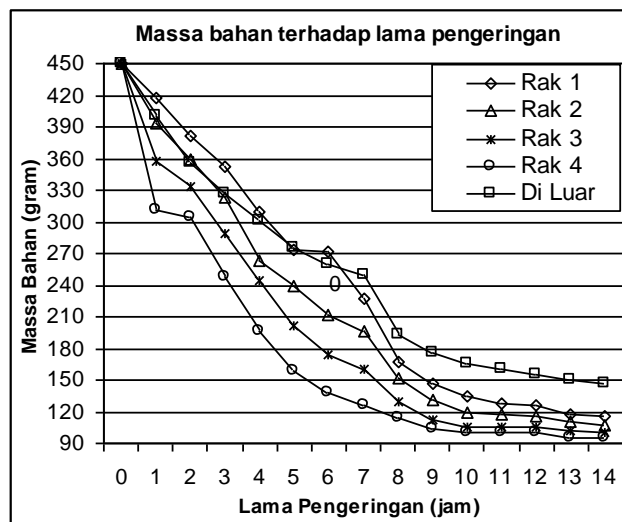
Gambar 4.1 Pengurangan Massa bahan yang dikeringkan terhadap waktu pengeringan
