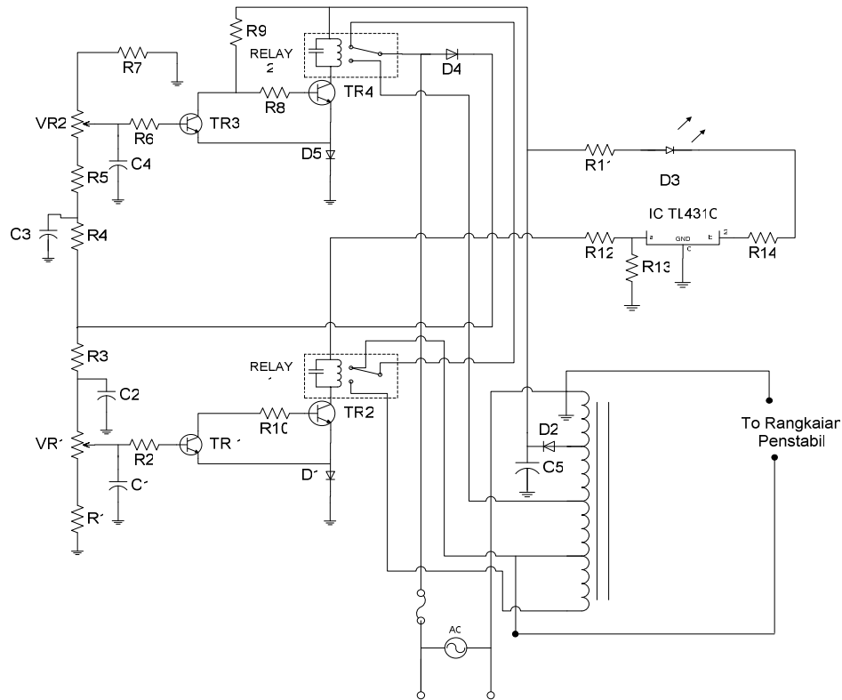
Gambar 4. Rangkaian Kontrol
