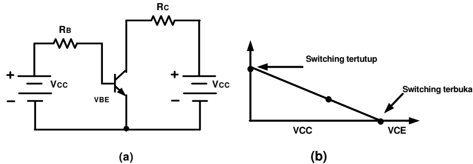
Gambar 1 (a). Karakteristik Statis Transistor. (b). Garis Beban dc (Malvino, 1994)
