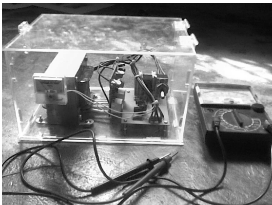
Gambar 6. Gambar alat penstabil tegangan bolak – balik satu fasa 220 V, 50 Hz menggunakan thyristor dengan daya 1, 5 kVA
