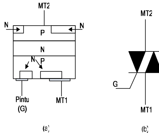
Gambar 2. (a) Struktur bangunan triac. (b) Lambang triac. (Wasito, 1990)
