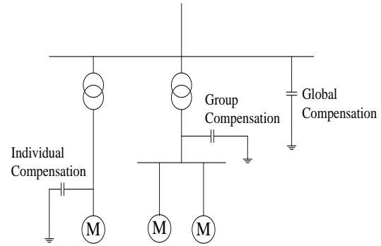
Gambar 7. Metode Pemasangan Instalasi Kapasitor Bank
