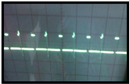
Gambar 13. Keluaran Detektor Fasa Satu Motor dan Satu Kapasitor
