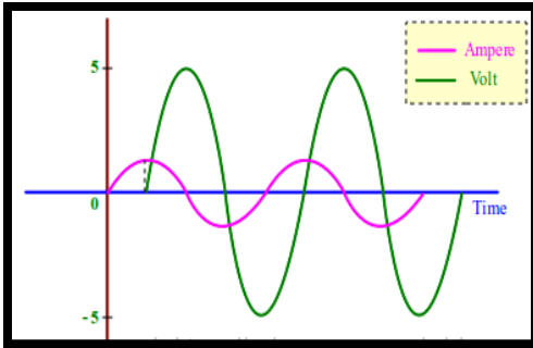
Gambar 6. Beban Kapasitif
