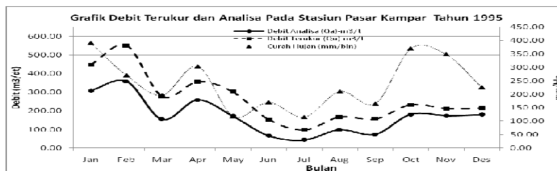
Gambar 6. Grafik Hubungan Debit Terukur dan Debit Analisa Tahun 1995 Pada Stasiun Pasar Kampar
