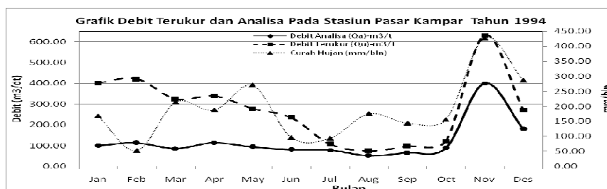
Gambar 5. Grafik Hubungan Debit Terukur dan Debit Analisa Tahun 1994 Pada Stasiun Pasar Kampar
