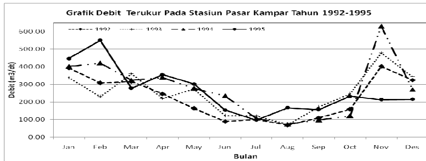
Gambar 7. Grafik Debit Terukur Tahun 1992-1995 Pada Stasiun Pasar Kampar
