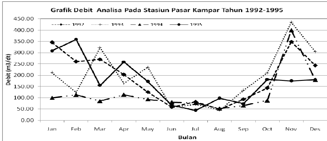
Gambar 4.7. Grafik Debit Analisa Tahun 1992-1995 Pada Stasiun Pasar Kampar
