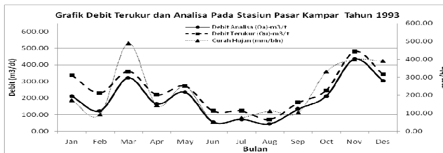
Gambar 4. Grafik Hubungan Debit Terukur dan Debit Analisa Tahun 1993 Pada Stasiun Pasar Kampar.
