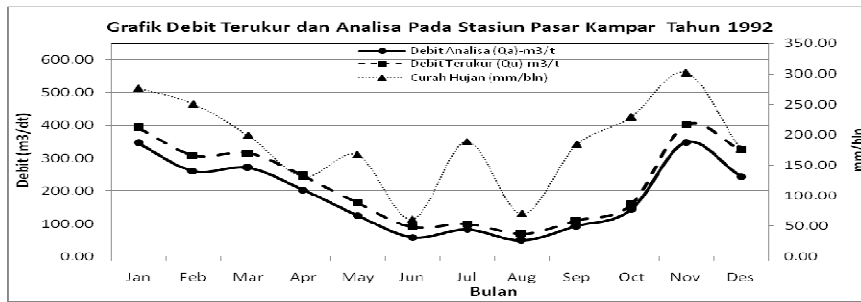
Gambar 3. Grafik Hubungan Debit Terukur dan Debit Analisa Tahun 1992 Pada Stasiun Pasar Kampar
