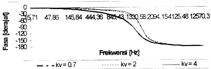
Gambar 4 (b) Gambar 4 (a) (b). Bode plot Magnitude dan Fasa dari G(s), dengan nilai gain K_v yang berbeda
