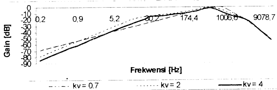
Gambar 5. Bode plot F(s), fungsi alih loop tertutup antara keluaran dan disturbed
