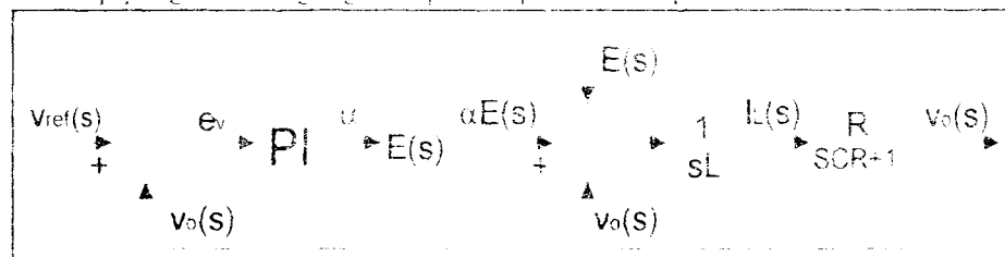
Gambar 2. Diagram Blok Chopper PWM Tegangan Terkendali
