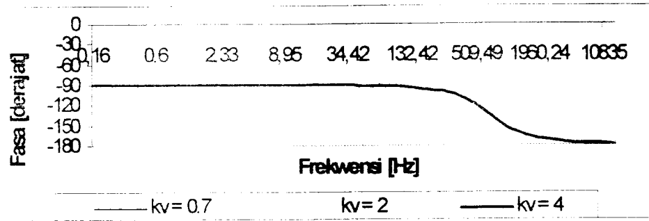
Gambar 3(b) Gambar 3 (a) (b). Bode Plot Magnitude dan Fasa dari T(s) dengan Nilai Gain Pengendali K_v yang Berbeda
